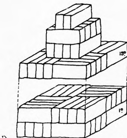
Figura 9 - Empilhamento do tijolo maciço
