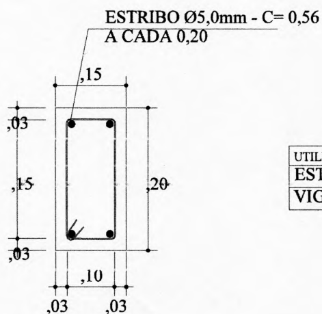
CORTE AA
