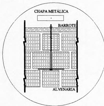
DETALHE DE AMARRAÇÃO DO BARROTE
